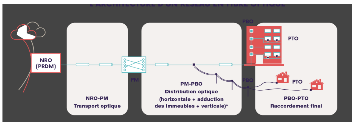
Schéma n° 3 : L'architecture d'un réseau de fibre optique
